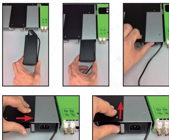
电源安装
