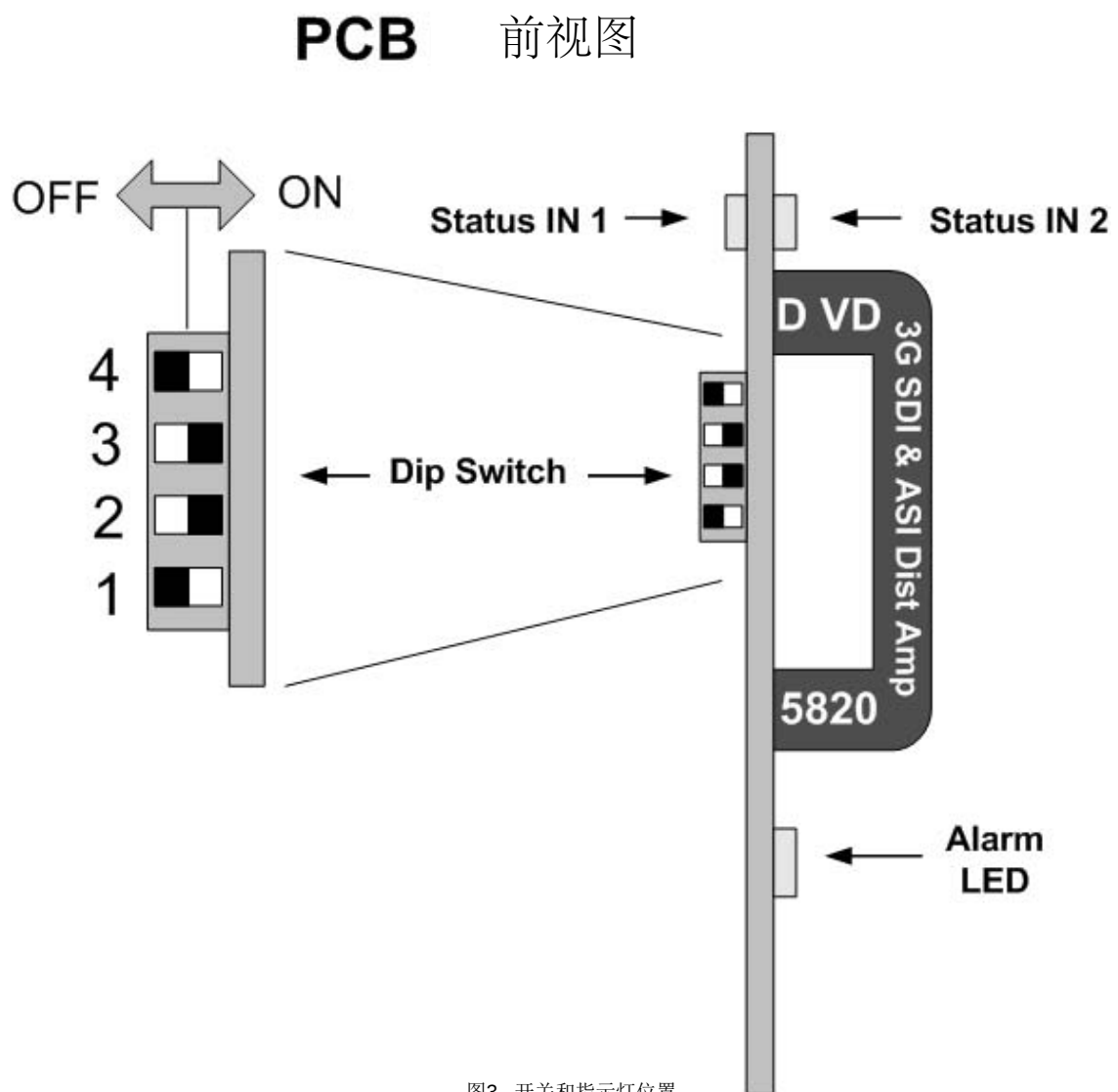
图3 -开关和指示灯位置
