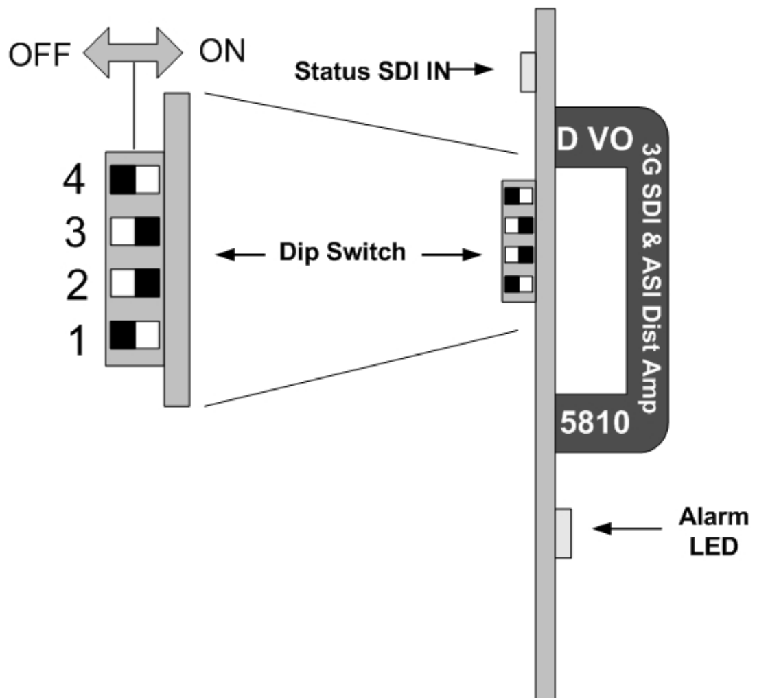
图3 -开关和指示灯位置
