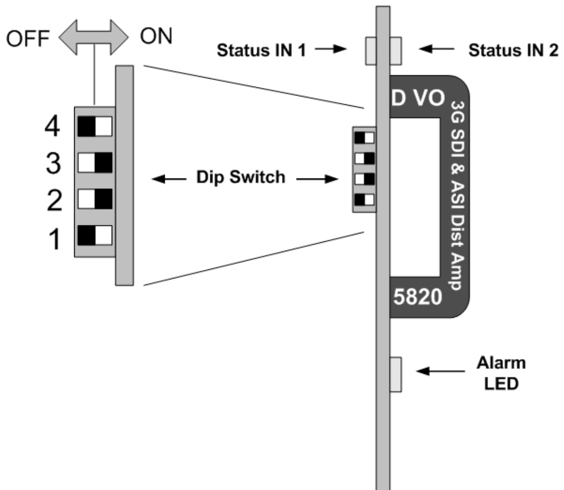
图3 -开关和指示灯位置
